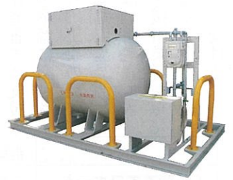
LPガス災害バルク貯槽 非常用発電機やGHP（ガスヒートポンプ）エアコンの動力エネルギーとして使われる
