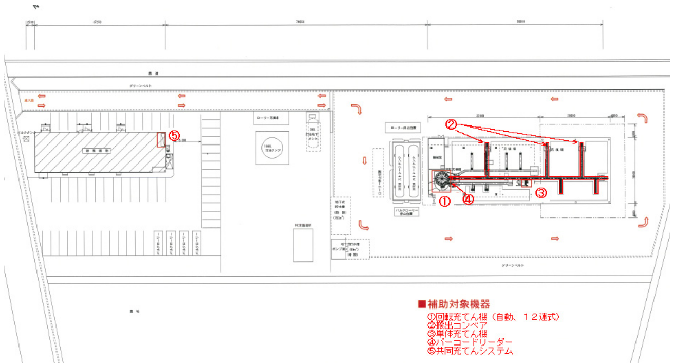
<図2>増強充てん所増強設備配置図
