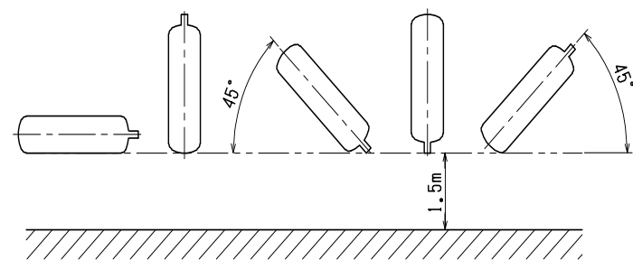
図 17.1 落下試験における落下姿勢（単位mm）
