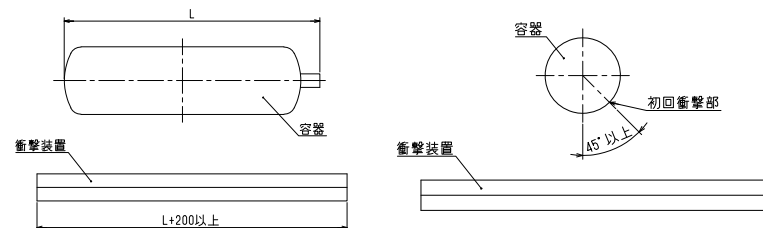
図 18.3 アングル衝撃試験の衝撃位置（単位mm）
