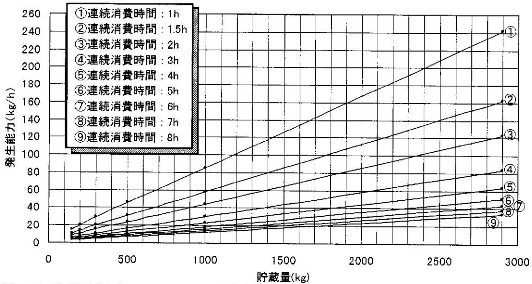
付図4.14 充填時組成 C_3H_8 : 90mol%, 残液量 : 50wt%, 地中温度 : 5°C, 充填時温度 : 5°C
