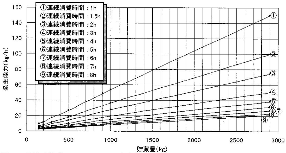
付図 4.8 充填時組成 C_3H_8 : 90mol%, 残液量 : 30wt%, 地中温度 : 5°C, 充填時温度 : 5°C
