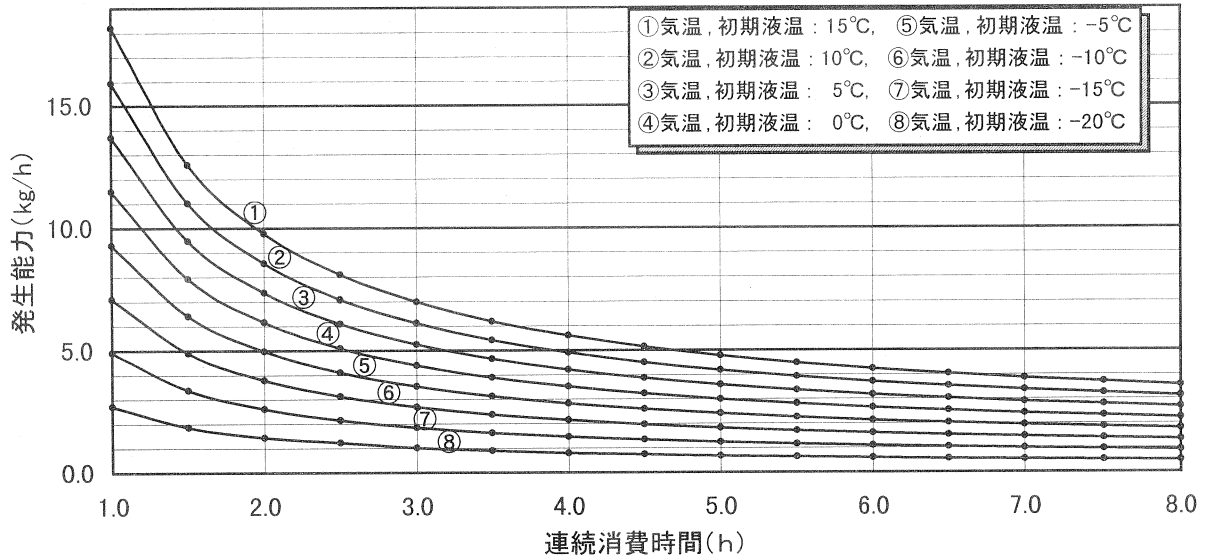
付図 1.22 200kg 型, 残液量 : 30wt%, 充填時組成 C_3H_8 : 95mol%
