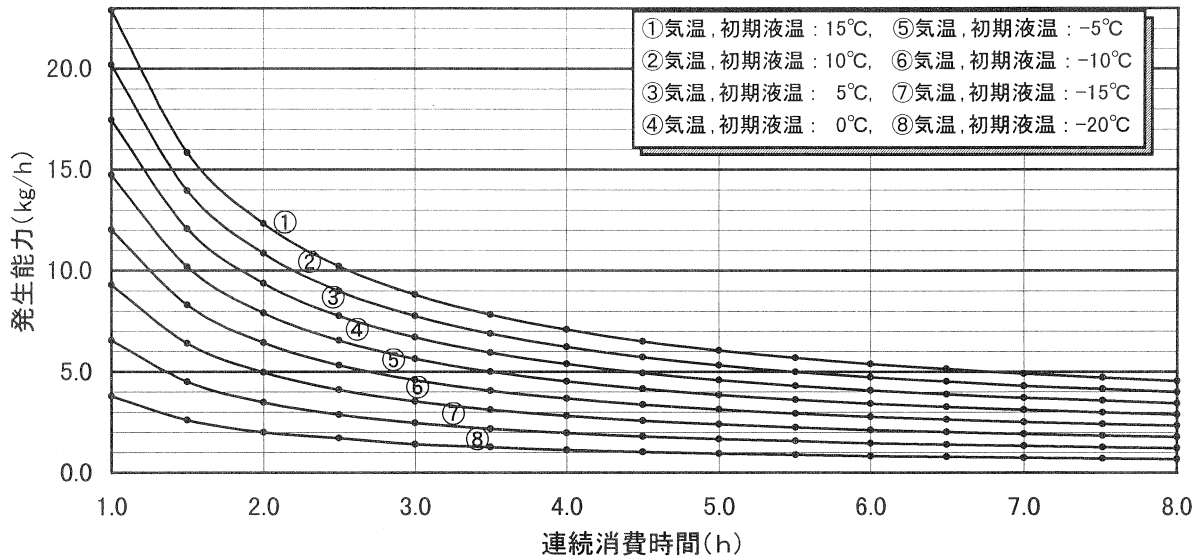
付図 1.25 200kg 型, 残液量: 40wt%, 充填時組成 C 3 H 8 : 95mol%
