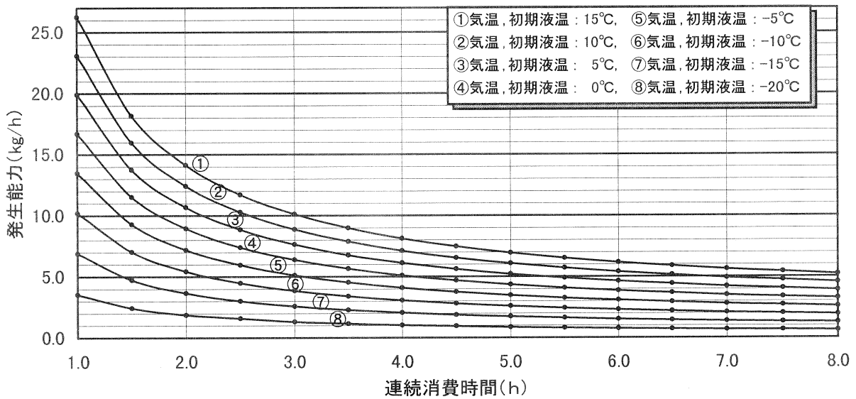
付図 1.29 200kg 型, 残液量 : 50wt%, 充填時組成 C_3H_8 : 90mol%
