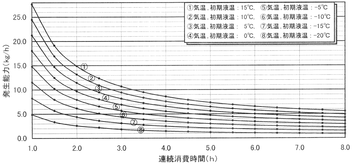
付図 1.28 200kg 型, 残液量 : 50wt%, 充填時組成 C_3H_8 : 95mol%
