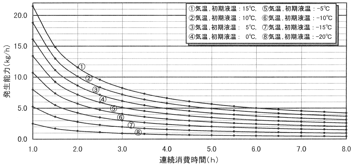
付図 1.26 200kg 型, 残液量: 40wt%, 充填時組成 C 3 H 8 : 90mol%
