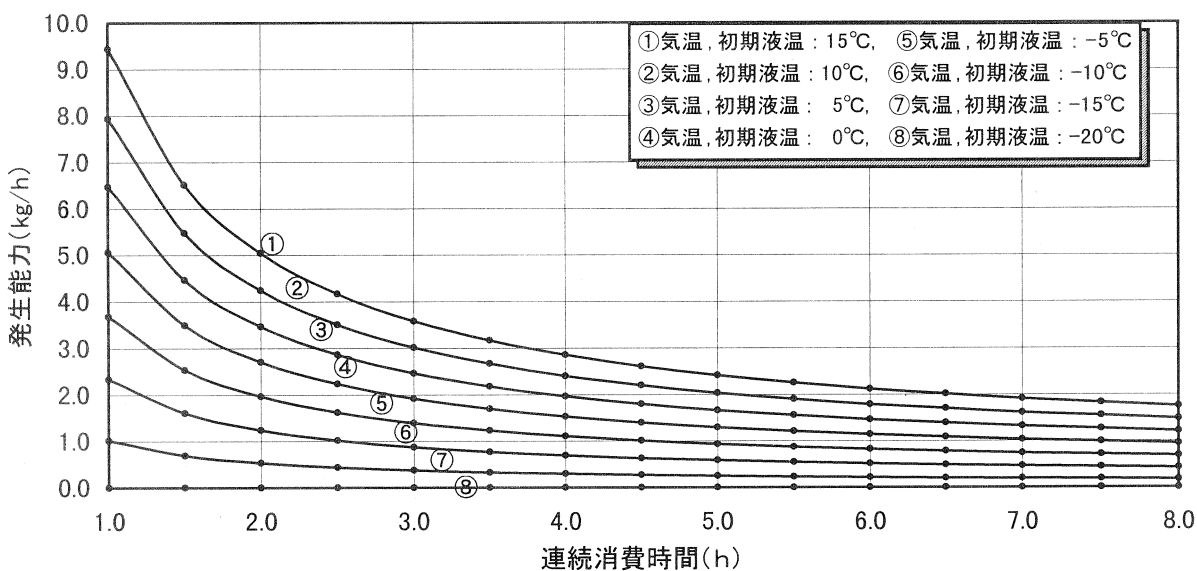
付図 1.17 200kg 型, 残液量 : 15wt%, 充填時組成 C_3H_8 : 90mol%
