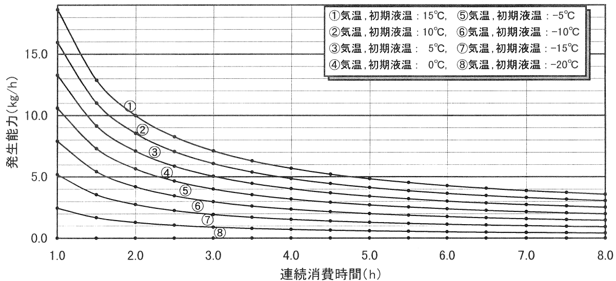
付図 1.27 200kg 型, 残液量: 40wt%, 充填時組成 C 3 H 8 : 80mol%
