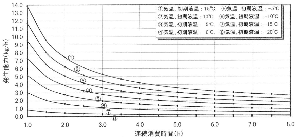
付 1.24 200kg 型, 残液量 : 30wt%, 充填時組成 C_3H_8 : 80mol%
