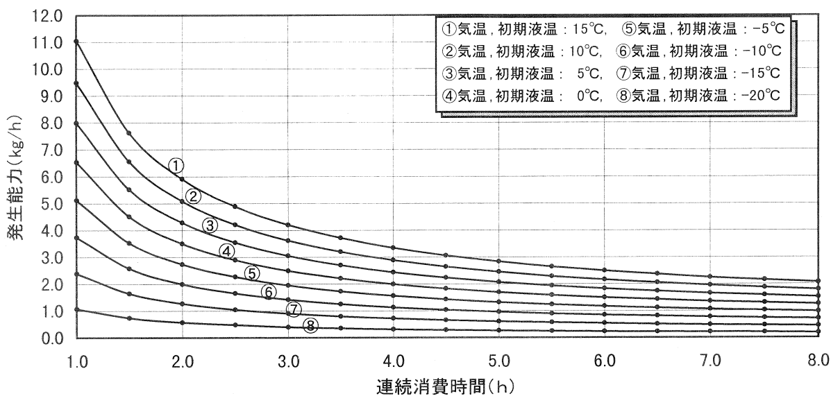
付図 1.16 200kg 型, 残液量 : 15wt%, 充填時組成 C_3H_8 : 95mol%
