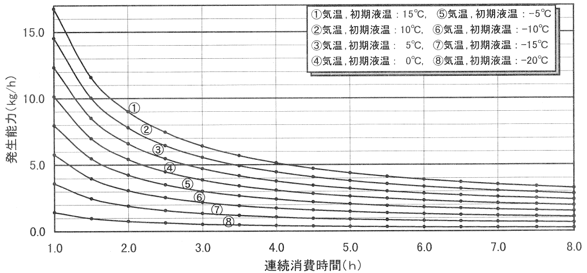
付図 1.23 200kg 型, 残液量 : 30wt%, 充填時組成 C_3H_8 : 90mol%
