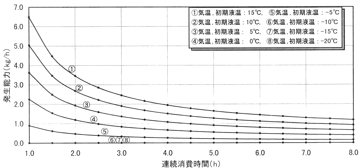
付図 1.18 200kg 型, 残液量 : 15wt%, 充填時組成 C_3H_8 : 80mol%
