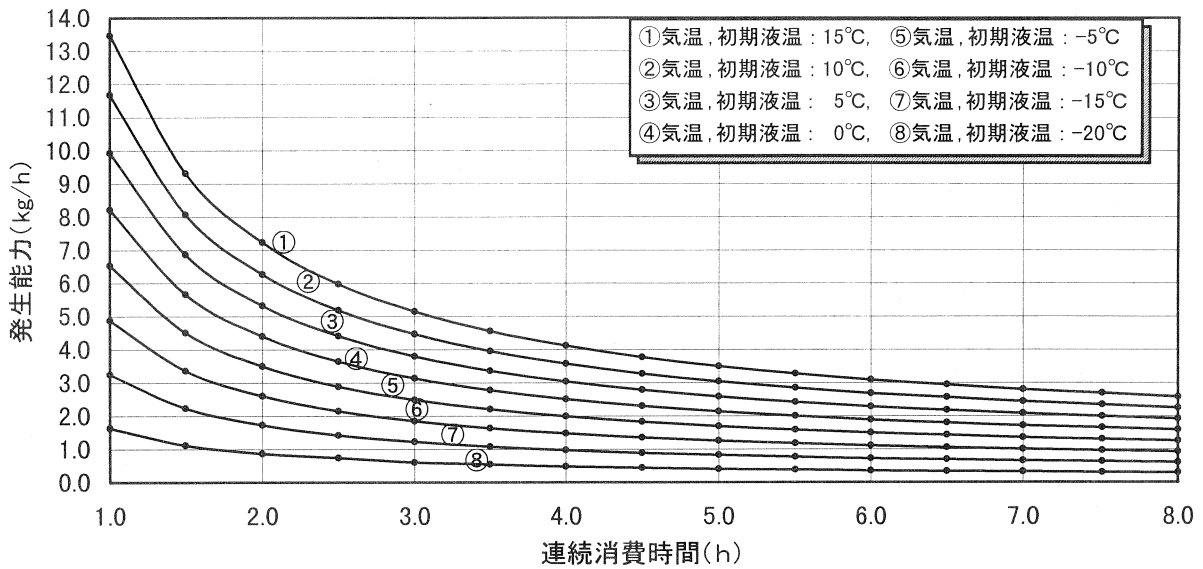
付図 1.19 200kg 型, 残液量 : 20wt%, 充填時組成 C_3H_8 : 95mol%
