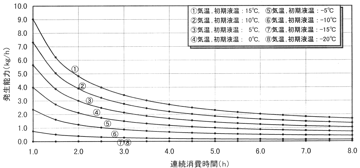
付図 1.21 200kg 型, 残液量 : 20wt%, 充填時組成 C_3H_8 : 80mol%
