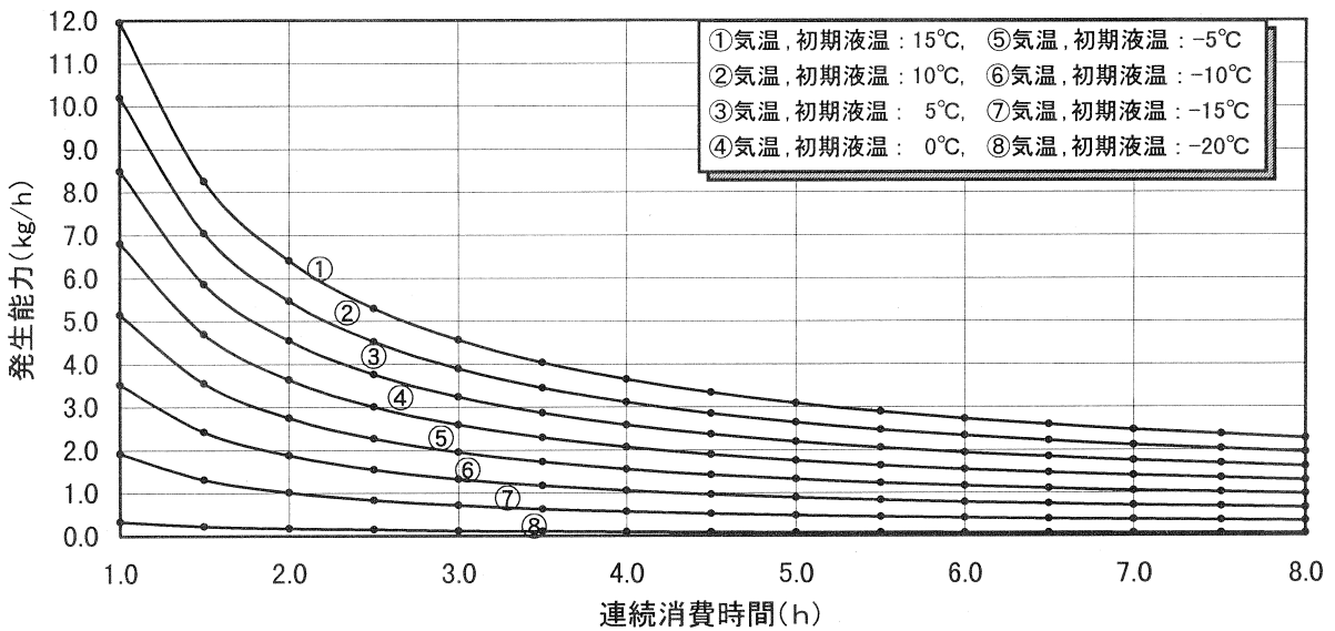
付図 1.20 200kg 型, 残液量 : 20wt%, 充填時組成 C_3H_8 : 90mol%
