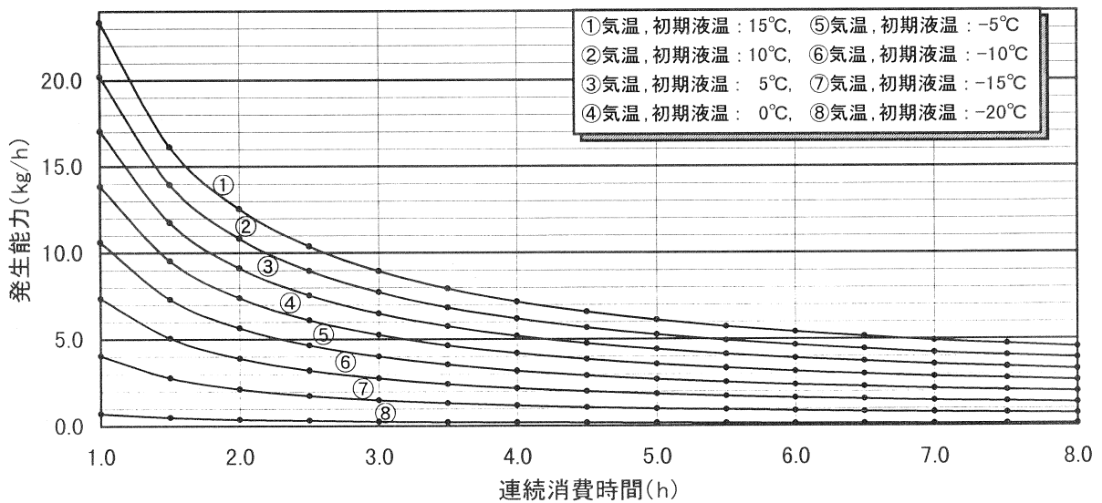
付図 1.30 200kg 型, 残液量 : 50wt%, 充填時組成 C_3H_8 : 80mol%
